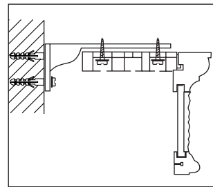
К стене, на шине
